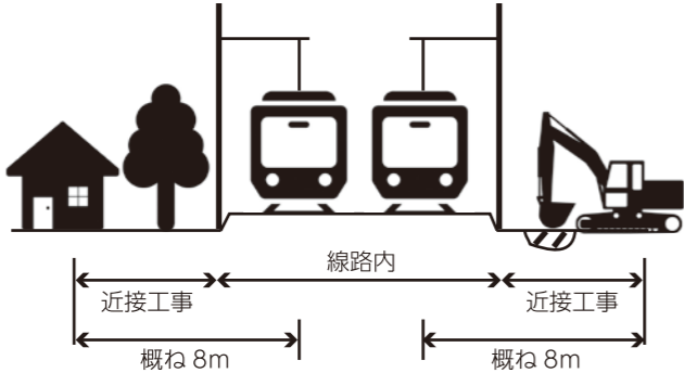
※作業内容や環境条件、使用重機によっては8m以上の場合でも近接工事の適用となる場合があります
