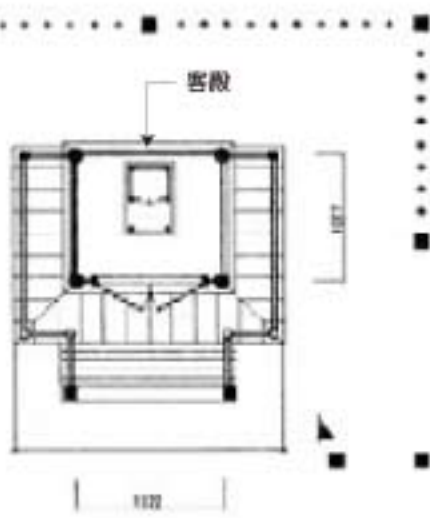
古野神社本殿平面図
