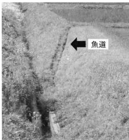
田んぼ(右上)と水路(左)をつなぐように設置された魚道(兵庫県豊岡市)
