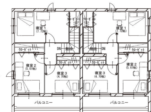
2階平面図 S=1/100
