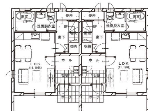
1階平面図 S=1/100
